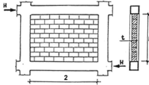
Interazione fra telai e pannelli murari di tamponatura Figura 1
