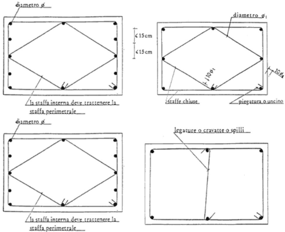
Indicazioni costruttive per strutture in calcestruzzo armato
