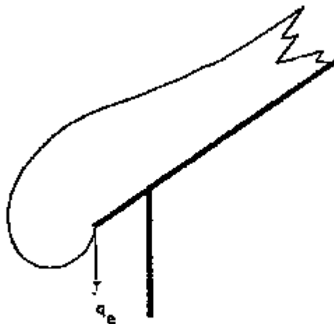
Fig. C.6.10 - Neve sporgente all'estremità di una copertura
