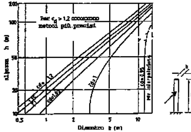
Fig. C.7.11 (a) - Ciminiere in acciaio, saldate, senza rivestimento interno.
