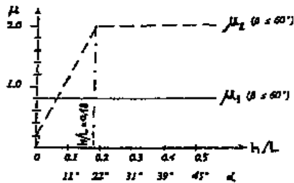
Fig. C.6.7 - Coefficienti di forma per differenti valori del rapporto altezza/lunghezza.
