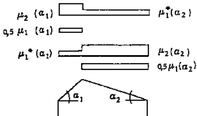
Fig. 6.4 - Condizioni di carico per coperture a due falde.
