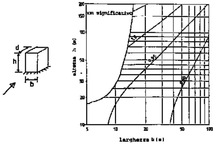
Fig. C.7.10 (c) - Edificio a struttura composta acciaio-calcestruzzo o edifici in acciaio con travi composte.
