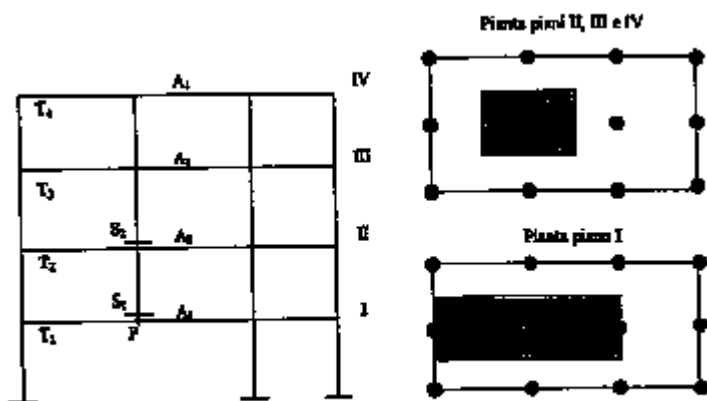
Fig. C.5.2 - Esempi schematici di individuazione dell'area di spettanza per la determinazione del coefficiente di riduzione dei carichi.
