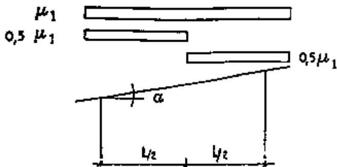
Fig. 6.3 - Condizioni di carico per coperture ad una falda.
