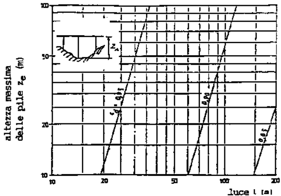
Fig. C.7.12 - Ponti stradali, ferroviari e pedonali
