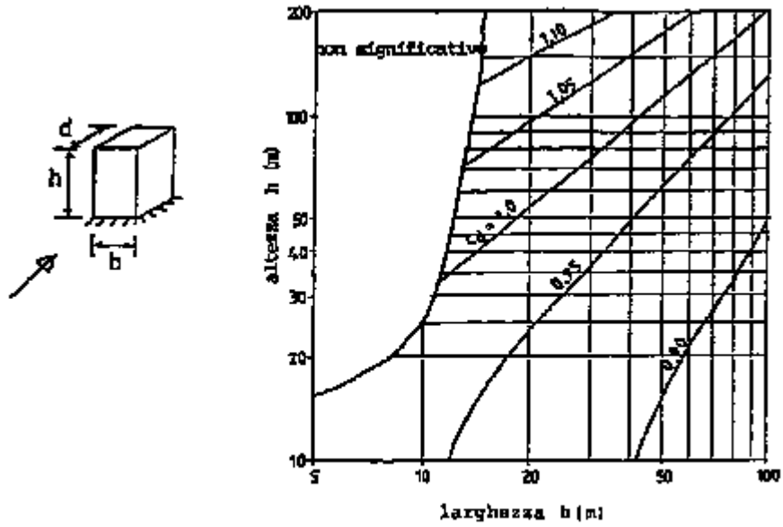
Fig. C.7.10 (b) - Edifici a struttura in acciaio.
