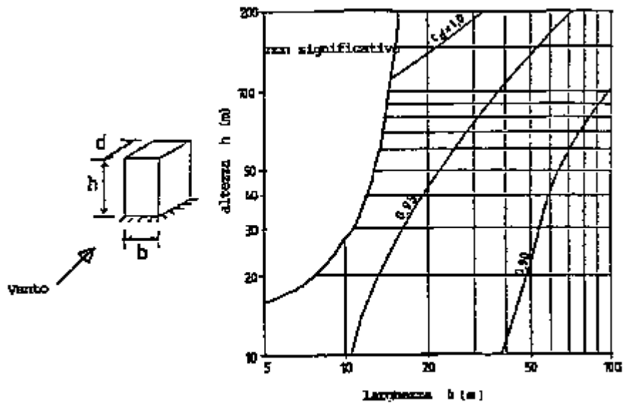
Fig. C.7.10 (a) - Edifici in cal. o in muratura.
