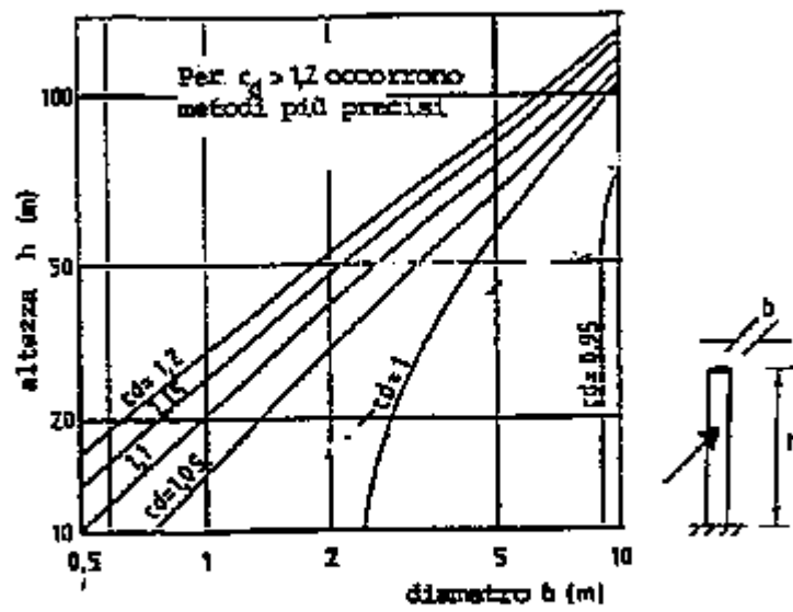
Fig. C.7.11 (b) - Ciminiere in acciaio, saldate, con rivestimento interno.
