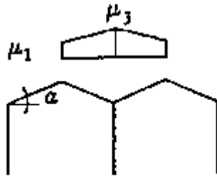
Fig. 6.5 - Condizione ulteriore di carico per coperture a più falde.
