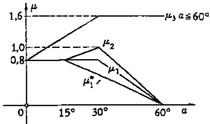
Fig. 6.2 - Coefficienti di forma per coperture a falde.
